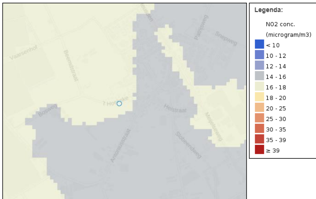
Figuur 19: Stikstofdioxide 2018 (Bron: Atlas leefomgeving)
