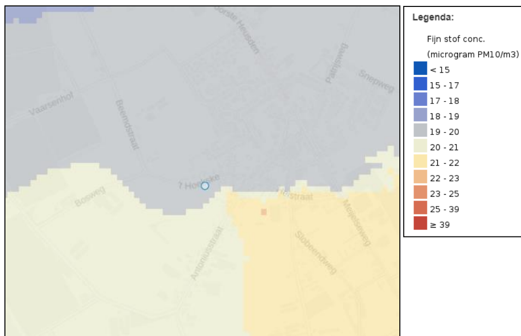
Figuur 17: Fijn stof PM 10 2019 (Bron: Atlas leefomgeving)
