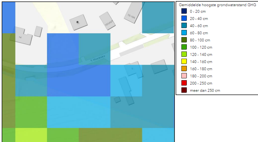
Figuur 10: Gemiddelde hoogste grondwaterstand
