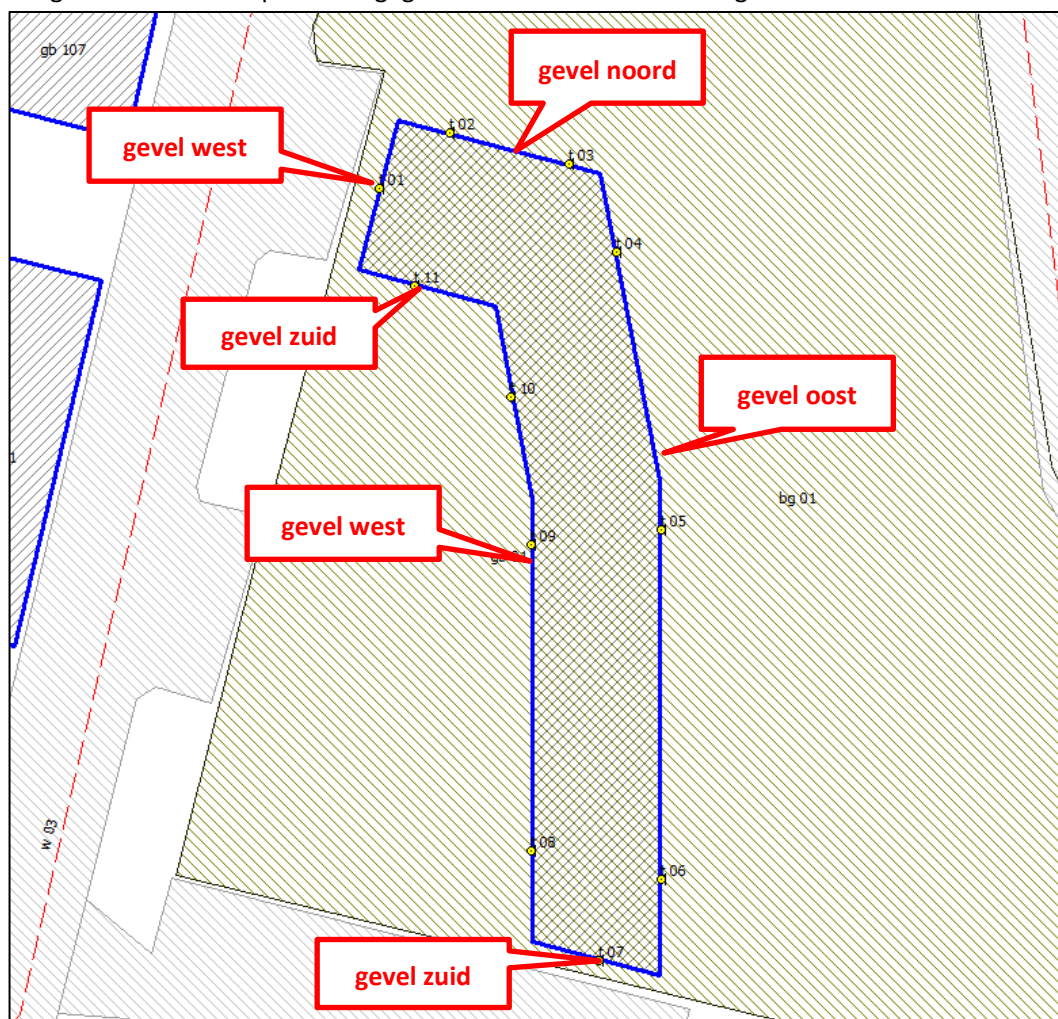
Figuur 2: Te toetsen gevels
